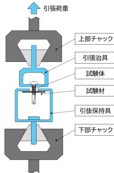
図3 単体引抜保持力試験方法
