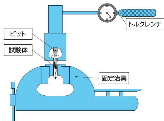
図2 単体ねじり強さ試験方法
