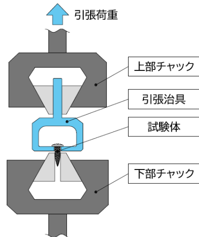
図1 単体引張破断試験方法
