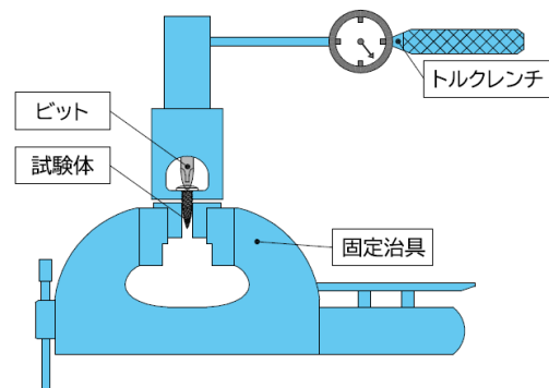
図2 単体ねじり強さ試験方法
