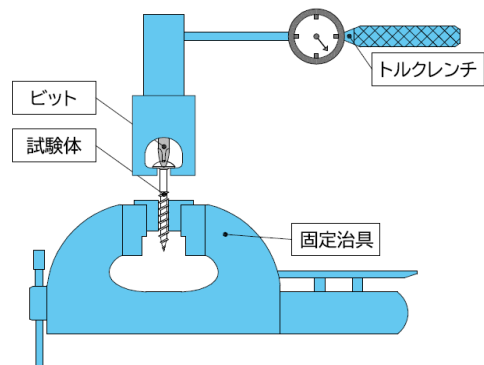
図2 単体ねじり強さ試験方法
