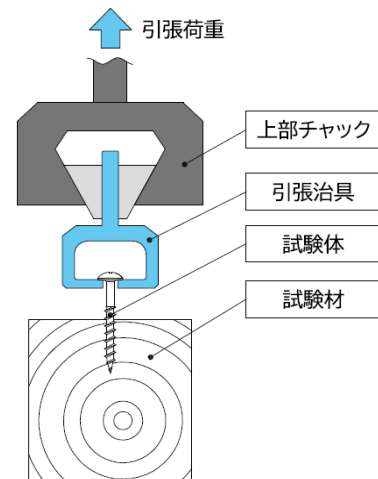
図3 単体引抜保持力試験方法
