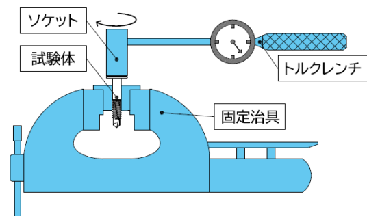
図2 単体ねじり強さ試験方法
