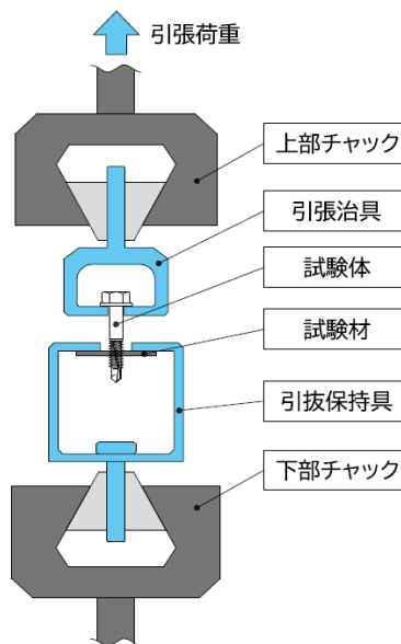
図3 単体引抜保持力試験方法
