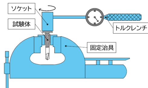
図2 単体ねじり強さ試験方法
