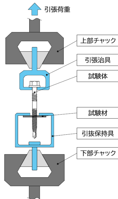
図3 単体引抜保持力試験方法
