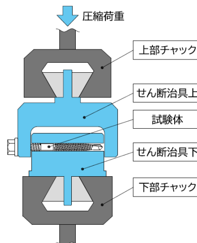
図4 単体せん断試験方法
