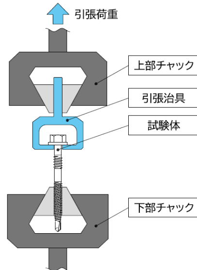
図1 単体引張破断試験方法
