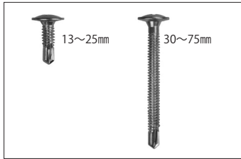
5mm径(マシンねじ首下テーパータイプ)
