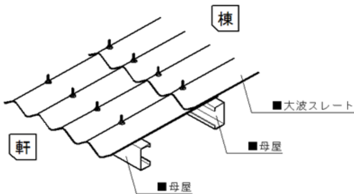
大波スレート 屋根イメージ図
